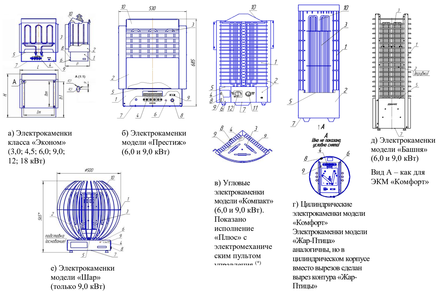
Рисунок 1 – Общие виды и устройство электрокаменок
