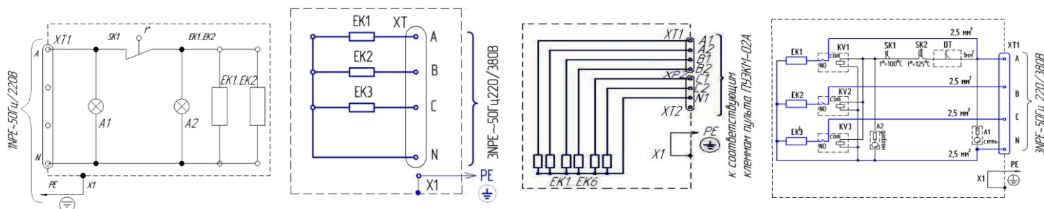
Рисунок 3 – Электрические схемы электрокаменок
